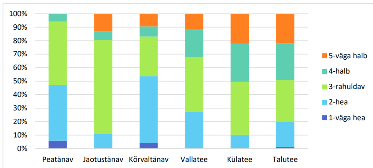
Joonis 22: Teekatte seisukord hinnatud aastal 2024 (allikas: Häädemeeste valla teehoiukava 2025-2029 )
